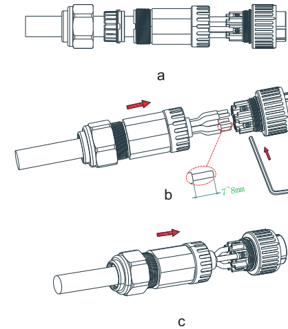
Kuva 6.2 AC-tuoton kytkentäkaavio
